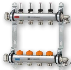
Dynacon Eclipse Durchflussbereich 30 - 300 l/h
