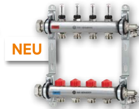
Dynacon 150 Durchflussbereich 10 - 170 l/h
